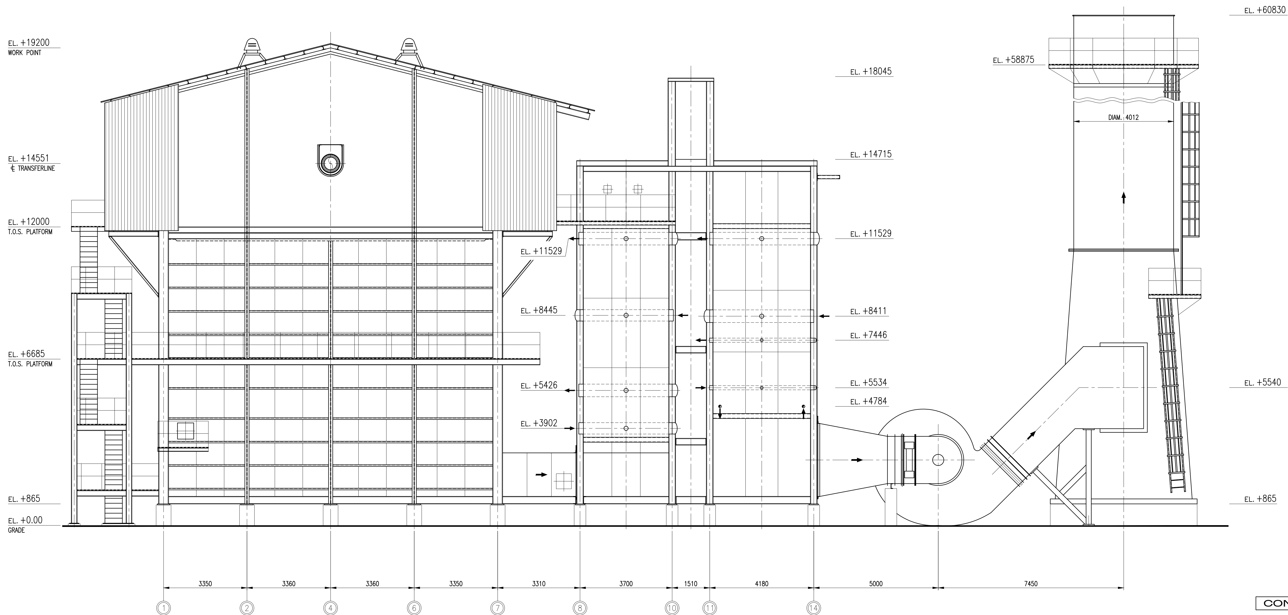
ELEVATION
